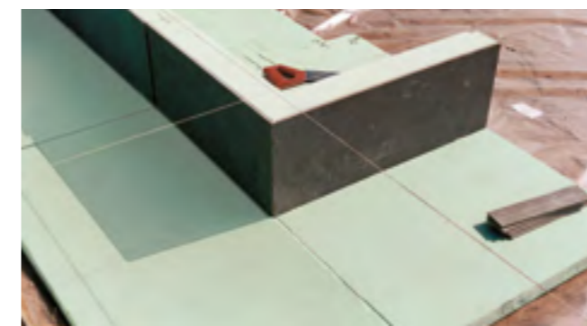
Fig. 3: Isolamento di una piastra di fondazione con Styrodur®.
