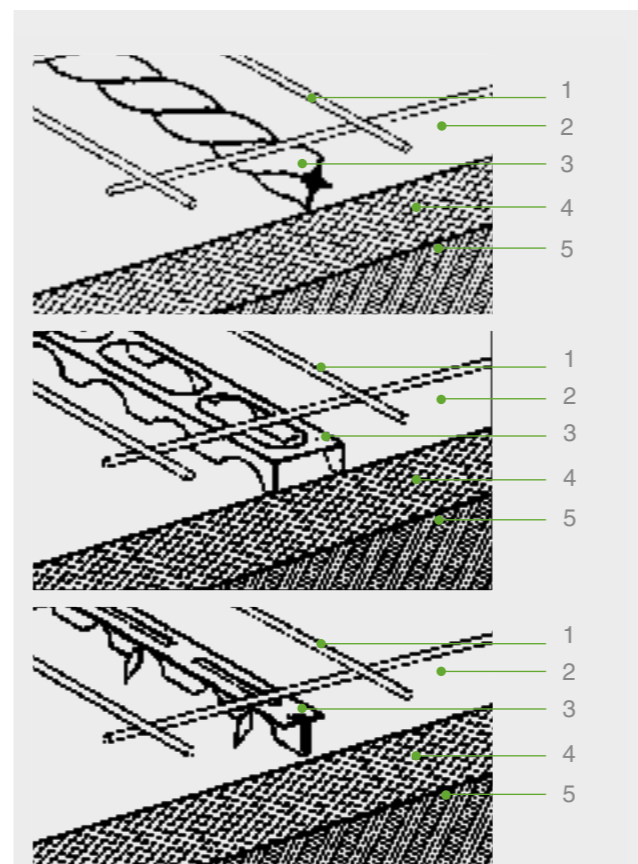
Fig. 10: Armatura posata sugli spessori.
