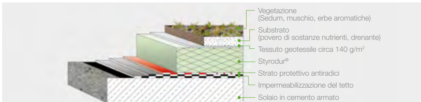
Fig. 25: sezione di un tetto rovescio rinverdito estensivamente.
