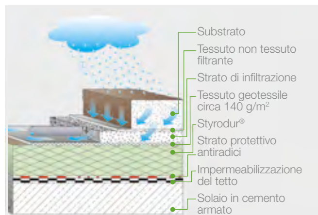
Fig. 30: Disposizione degli strati di un tetto rovescio verde con strato drenante per l'assorbimento superficiale dell'acqua e in alternativa con tubo drenante.
