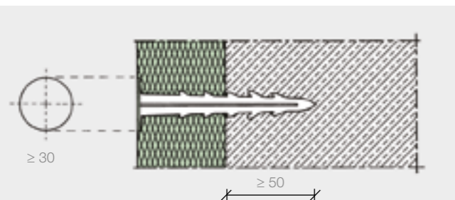
Fig. 15: Chiodi di plastica per l'ulteriore ancoraggio di Styrodur® 2800 C (misura in mm).
