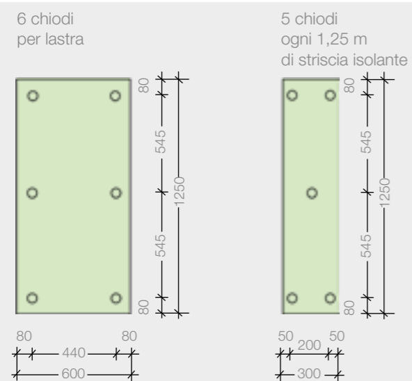
Fig. 16: Numero e disposizione possibili di chiodi di plastica per l'installazione di lastre di Styrodur® 2800 C nella cassaforma di calcestruzzo (misura in mm).
