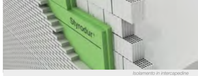
Isolamento in intercapedine
