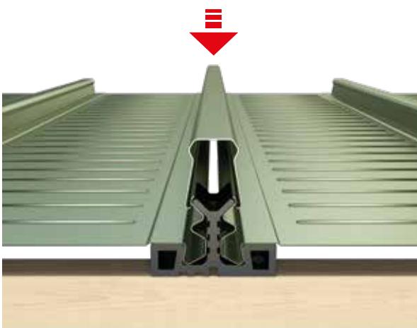
4 _ Applicazione cappello / Press down cap as shown
