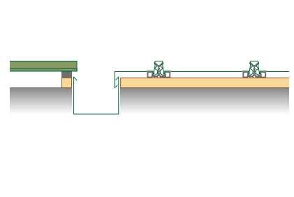
DETTAGLIO TECNICO TECHNICAL DETAIL
